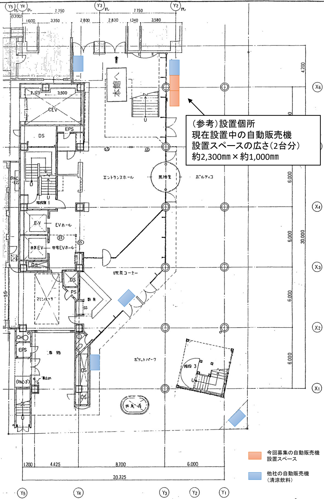
1階 平面図
